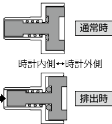
バルブ断面図
